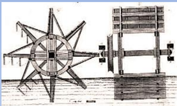
Водяное колесо и ходовой вал водяных колес 1 и 2 машинного водоходного судна
